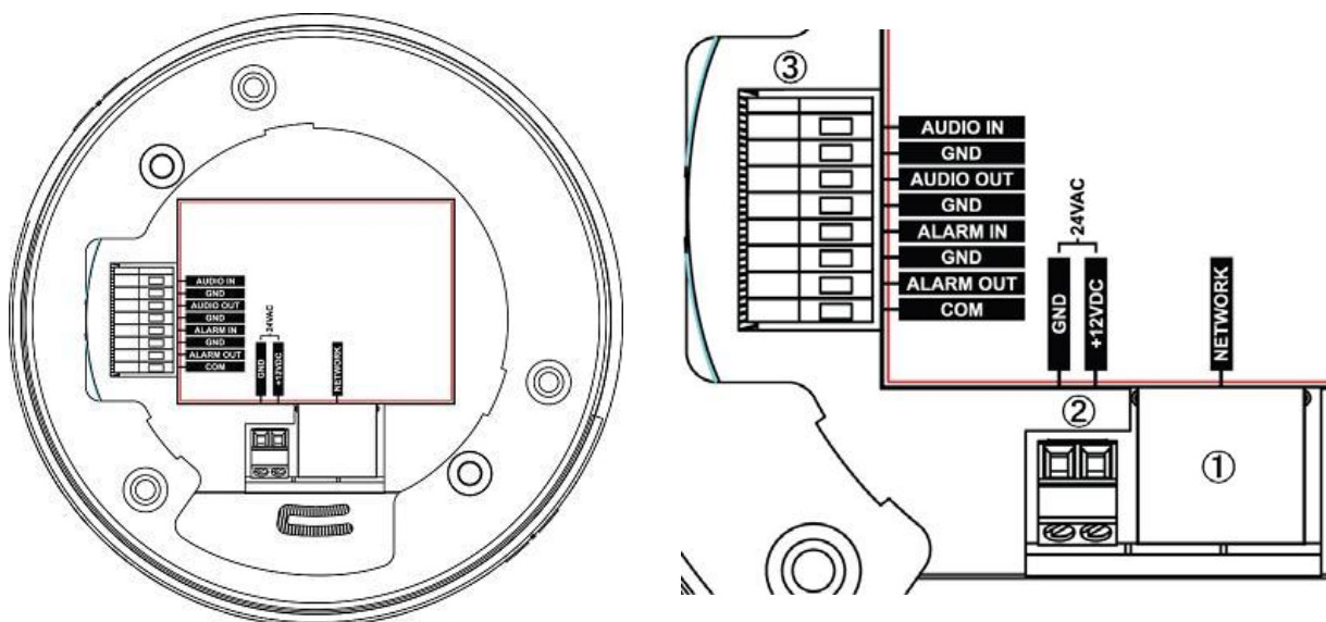
Рис.2.1. Задняя панель видеокмеры LTV-ICD*-723-V3.3-12
