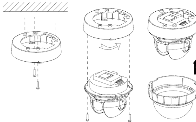
Рис.3.1. Подготовка к монтажу видеокамеры LTV-ICD*-723-V3.3-12
