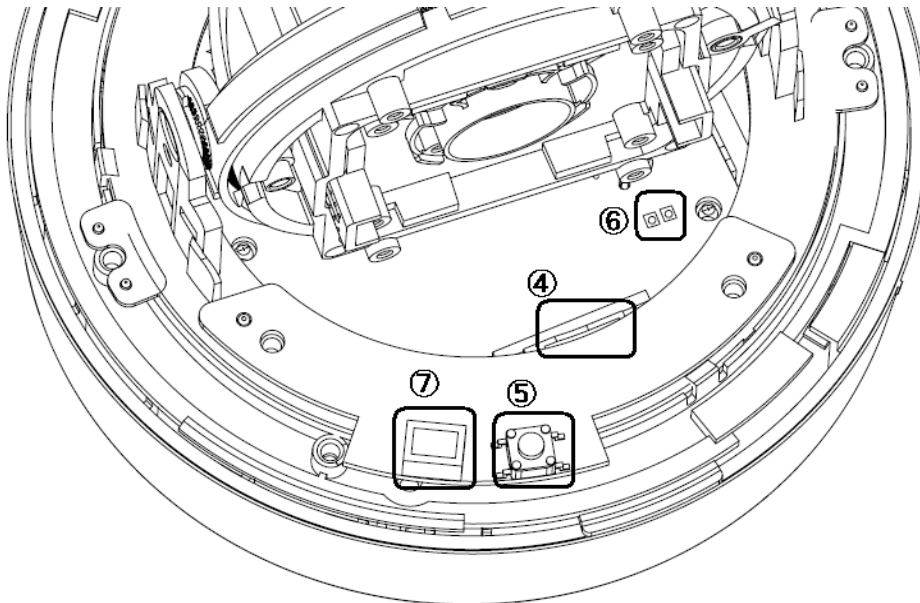
Рис.2.2. Разъемы видеокамеры LTV-ICD*-723-V3.3-12
