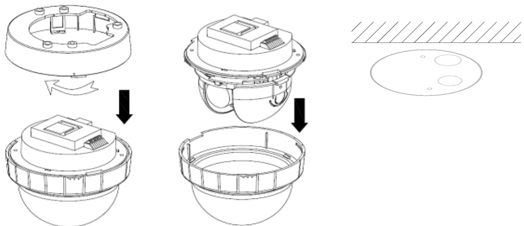
Рис.3.2. Монтаж видеокамеры LTV-ICD*-723-V3.3-12
