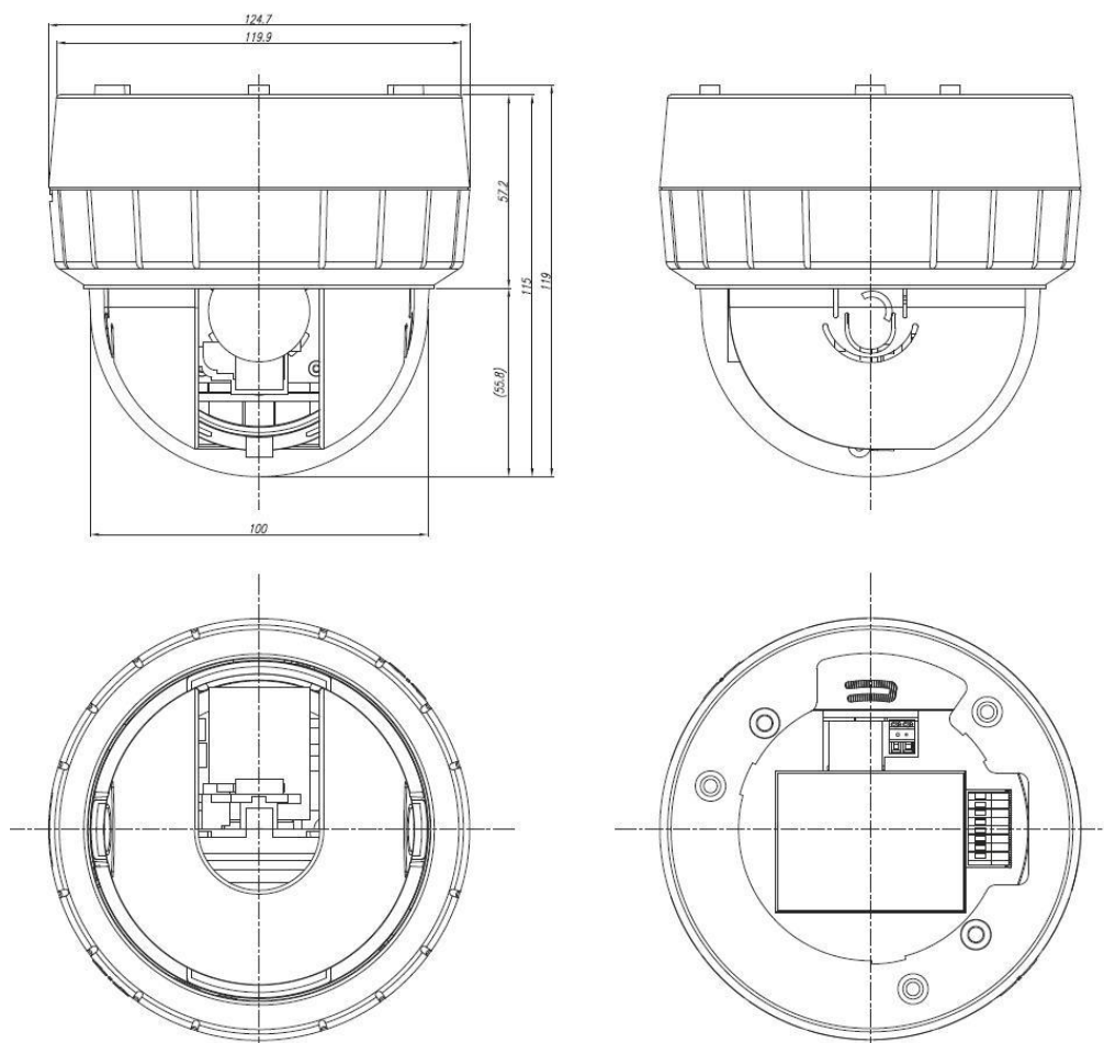
Рис.1.2. Габаритные размеры видеокамеры LTV-ICD*-723-V3.3-12
