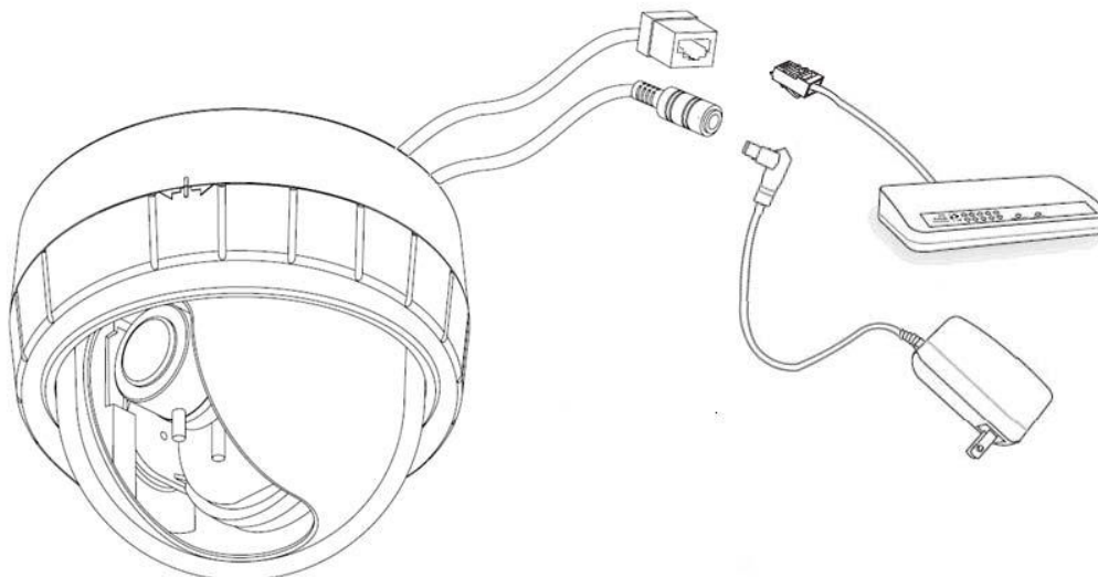
Рис.3.3. Подключение видеокамеры LTV-ICD*-723-V3.3-12
